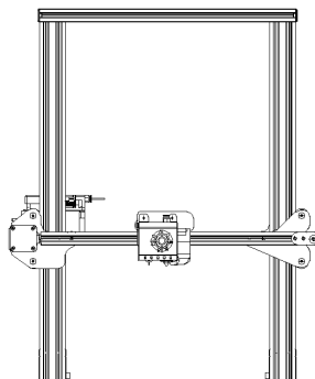
Gantry Frame
